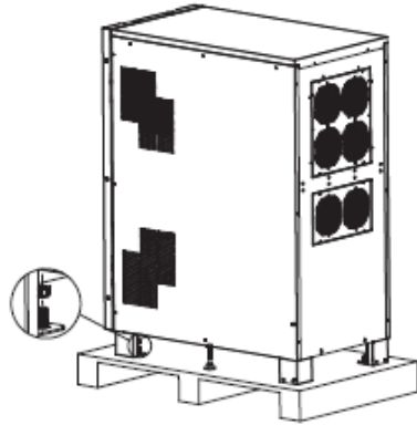
移除各个支撑脚的螺母
